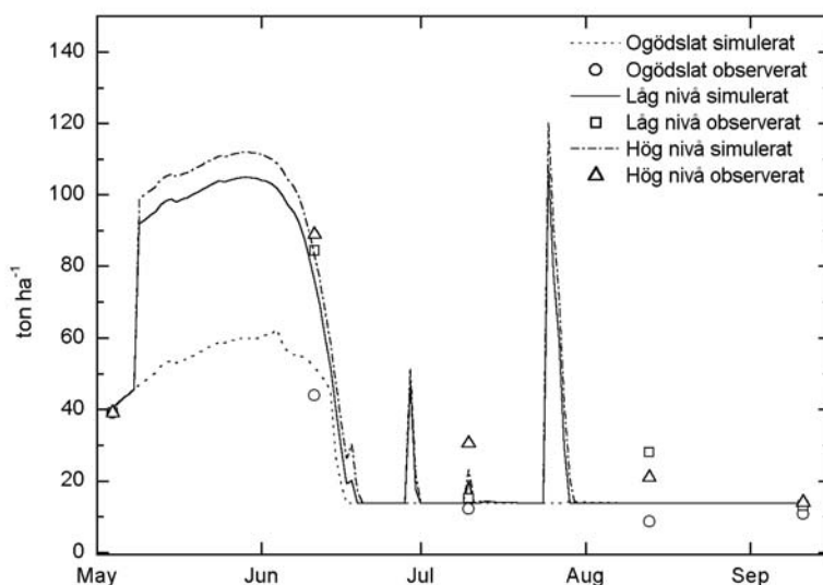
Figur 12. Mineralkväve i marken (0-30 cm), simulerat i N_ABLE (linjer) och efter provtagning och analys (symboler) för gödslad vitkål samt vid två olika tillförelsnivåer.
