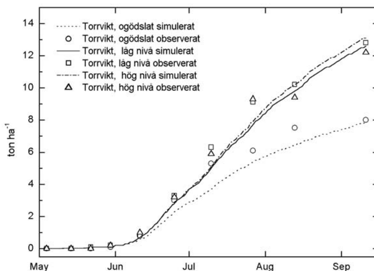
Figur 10. Torrsubstansvikt, simulerat i N_ABLE (linjer) och efter provtagning och analys (symboler) för ogödslad vitkål samt vid två olika tillförselnivåer.
