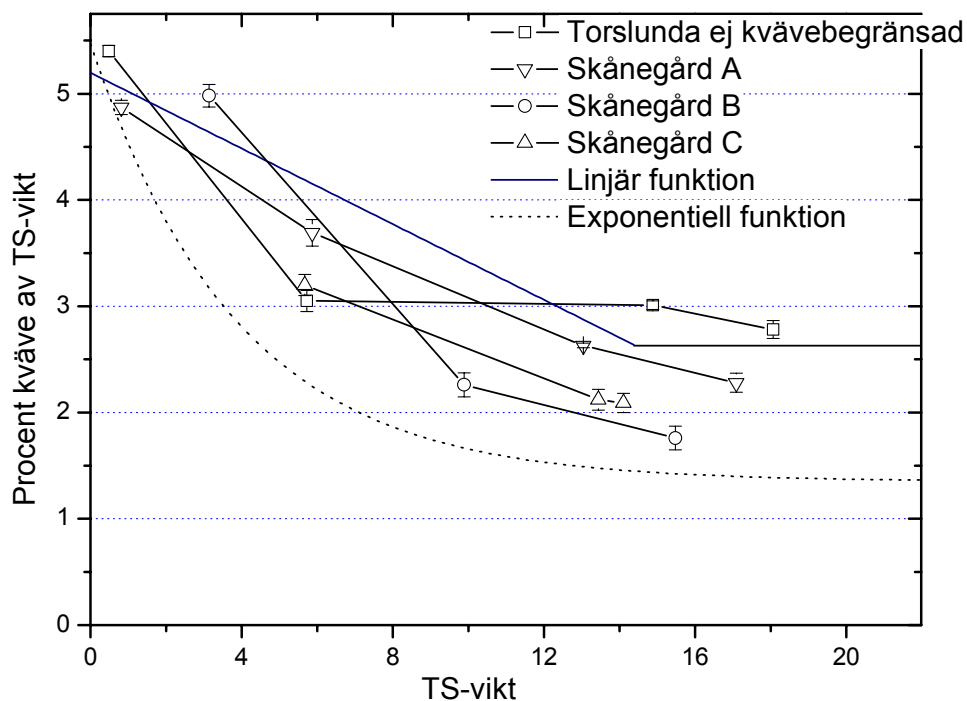
Figur 6. Koncentrationen av kväve i vitkål vid olika TS vikt i de kommersiella vitkålsfälten och i ej kvävebegränsad vitkål på Torslunda. Kurvor utan symbol anger varför minskningen i tillväxt inte verkar bero på kvävebrist.
