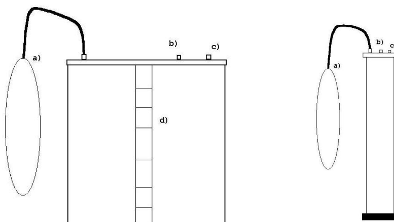
Bild 1. Till vänster visas pilotbehållaren (3 m 3 ) och till höger laboriekolonnen (30 l). a) är gasuppsamlingssäcken, b) är genomföring för gödselprovtagning, c) är membran för gasprovtagning och d) är ett siktglas.
