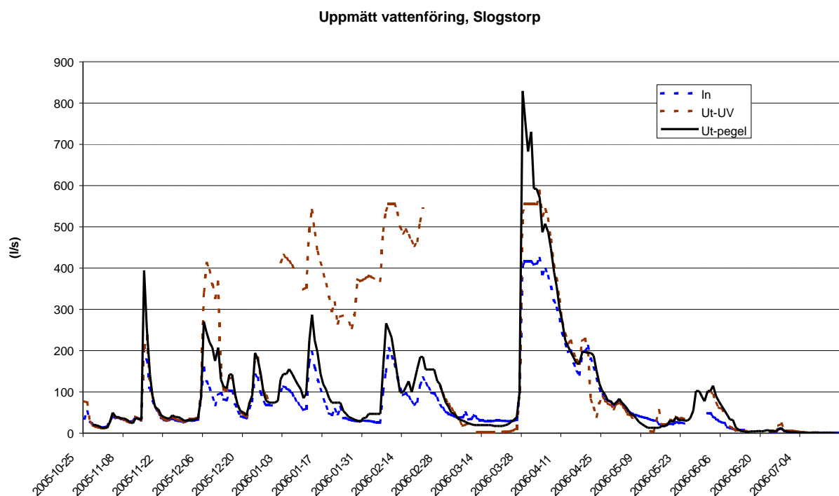
Figur 6. Uppmätt vattenföring i Slogstorp, med tryckgivare vid inloppet och med pegel respektive ultraljudsgivare (Ut-UV) vid utloppet. För In och Ut-UV visas kurvor som inte är kompenserade för ändrad utloppsreglering eller felaktig kalibrering (se text). Med hänsyn till dessa felregistreringar är överensstämmelsen generellt god mellan de tre kurvorna.
